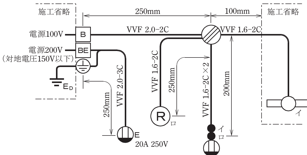
図1. 配線図
