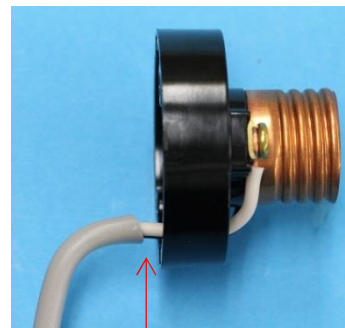
欠陥の例：ケーブル外装が台座の中に入っていない
