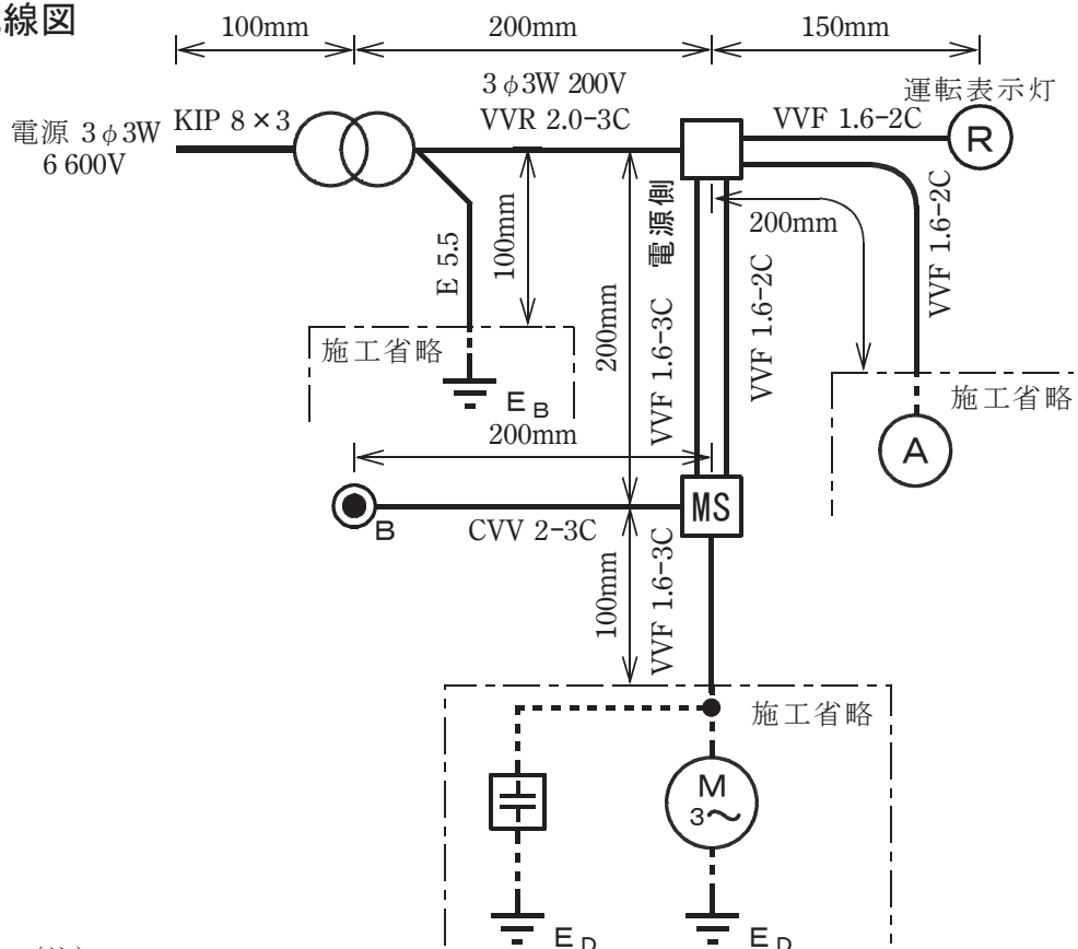
図1. 配線図
