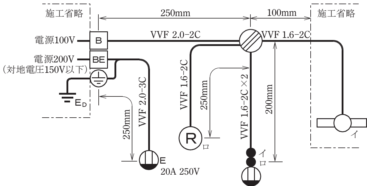
図 1. 配線図
