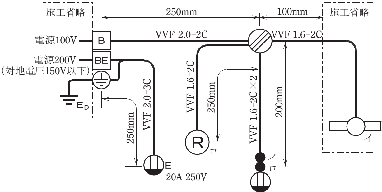
図 1. 配線図
