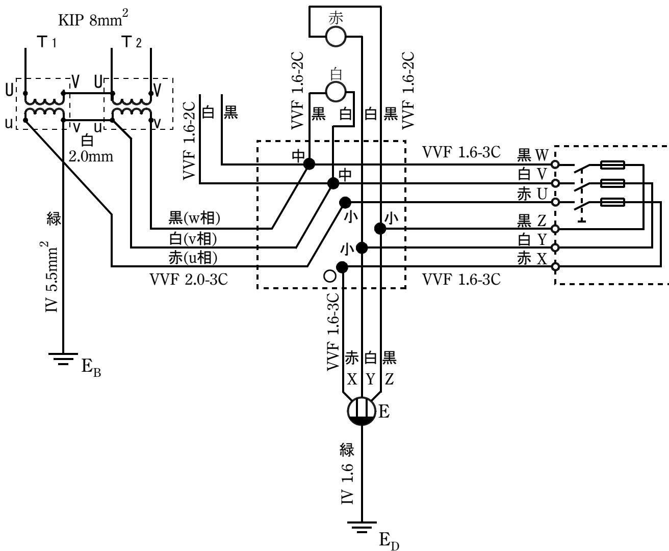
【複線図】
