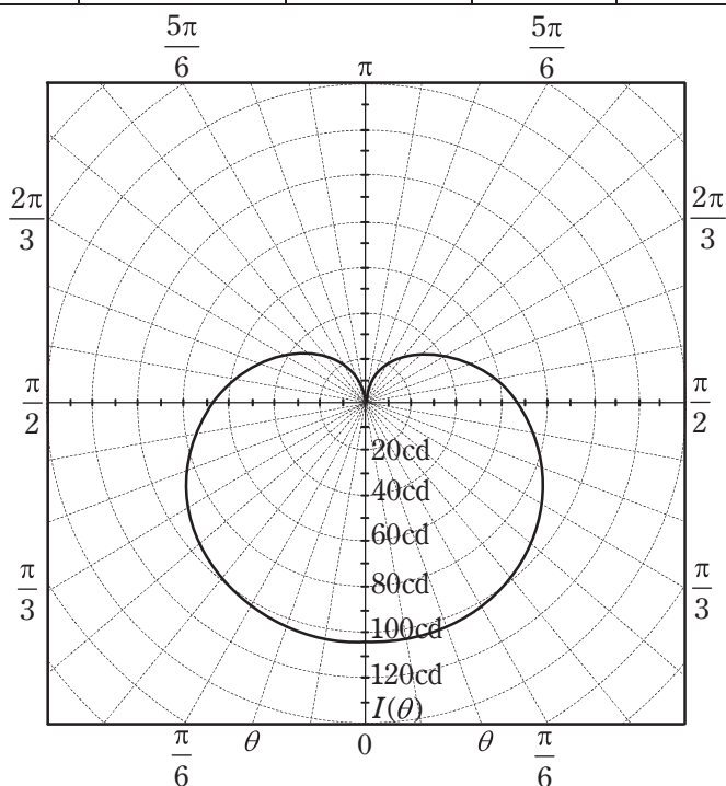
図 配光特性（鉛直角 \theta [rad] に対する光度 I(\theta) [cd] の分布）
