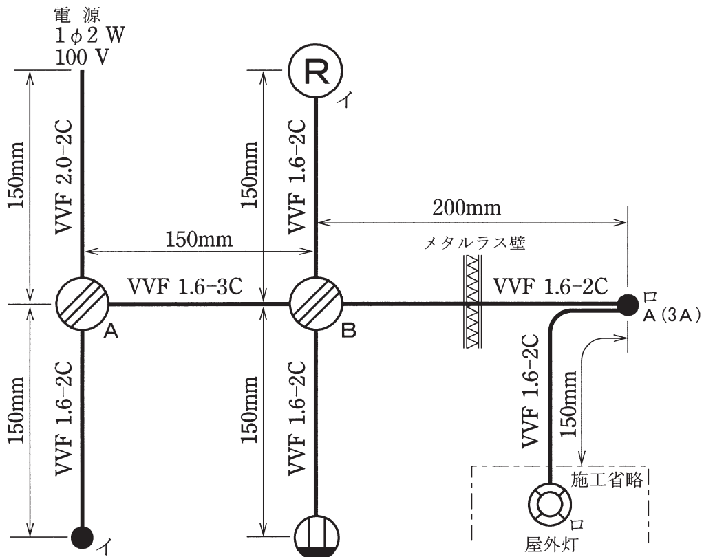
図1. 配線図
