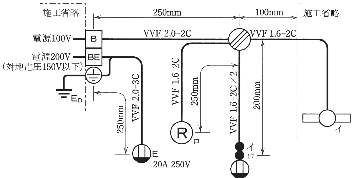
図1. 配線図
