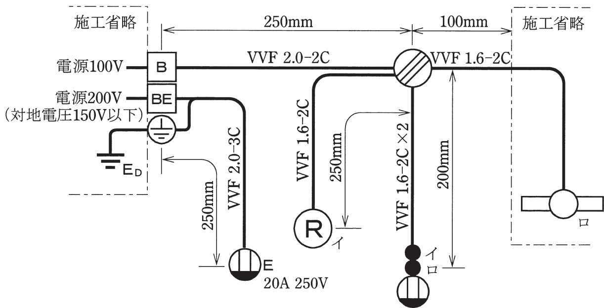
図1. 配線図
